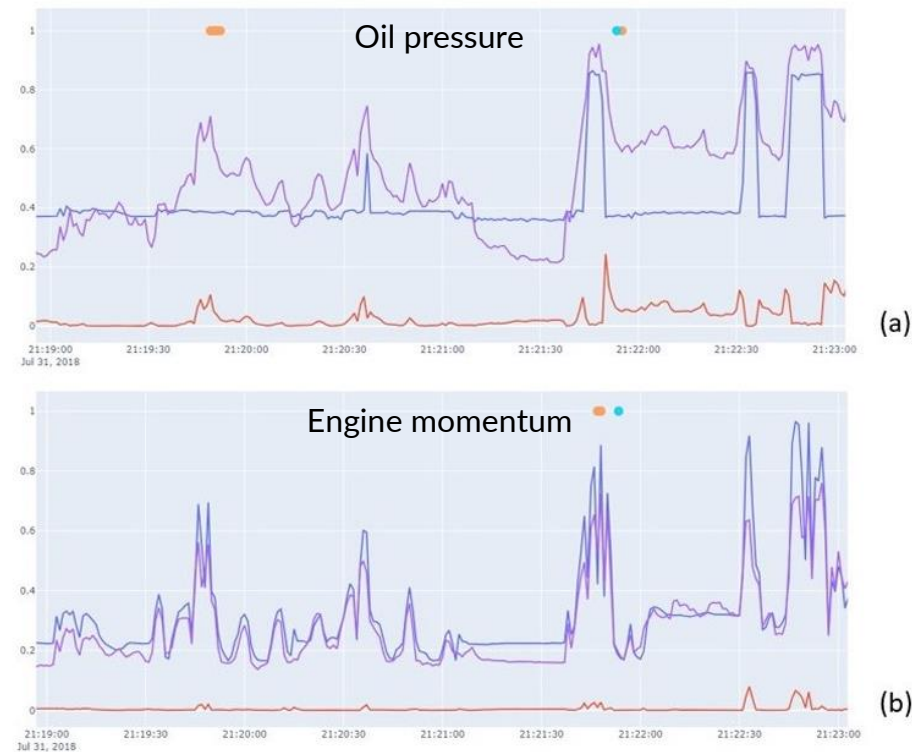
Détection d'une anomalie de pression d'huile moteur
